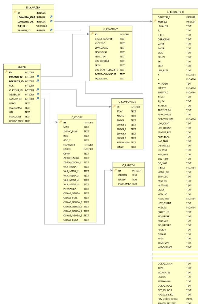
Obr. 1 | Schéma tabulek v datové bázi a jejich vazeb
